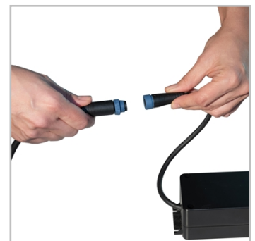
ILUM MARK utiliza conectores IP 68 de 2 pines (blanco) o 5 pines (RGB).
