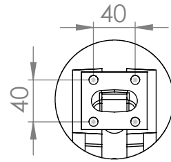
DETAIL A (LUMINAIRE INTERFACE)
